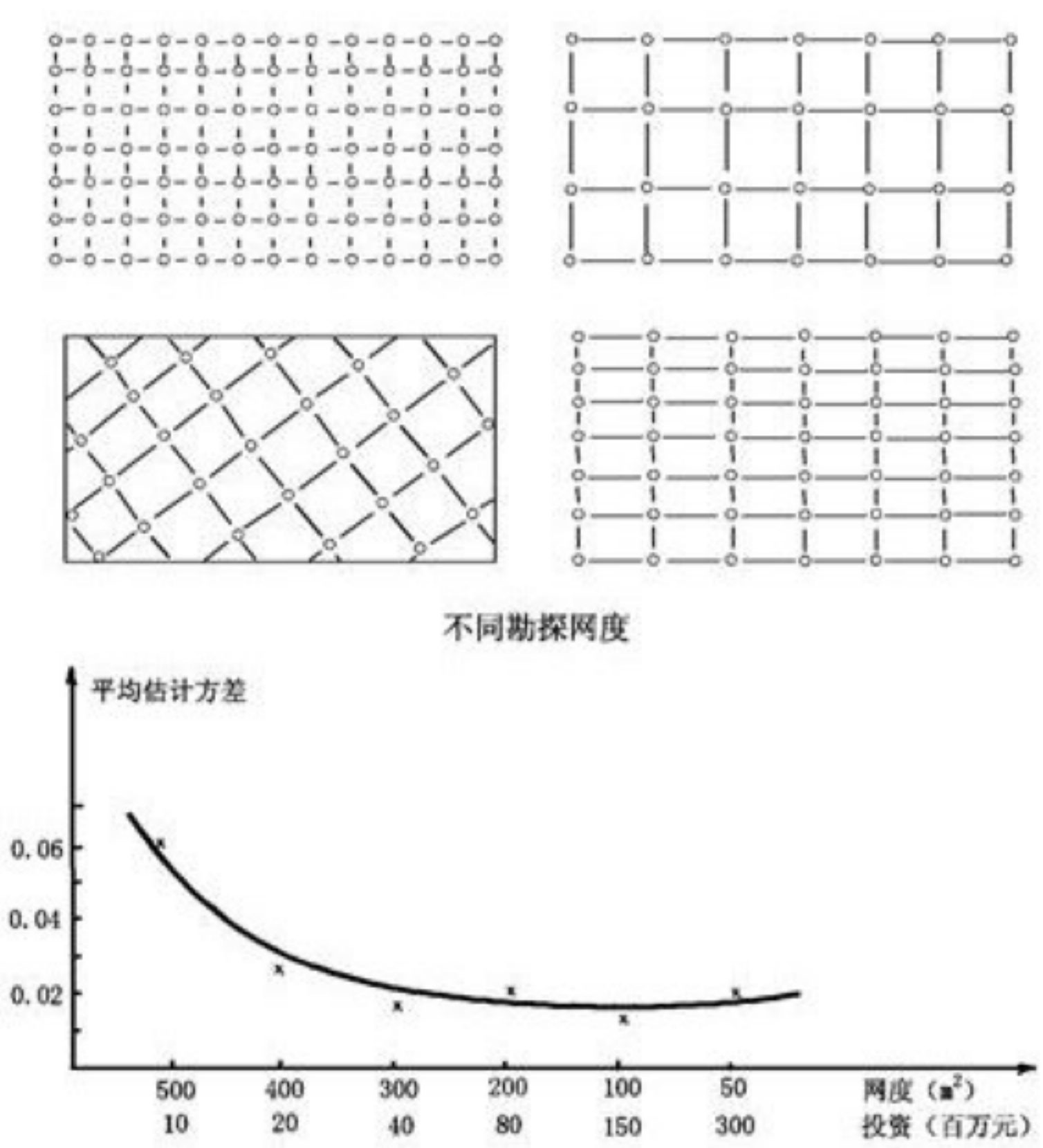
图 F.1 最优勘探网度的选择
