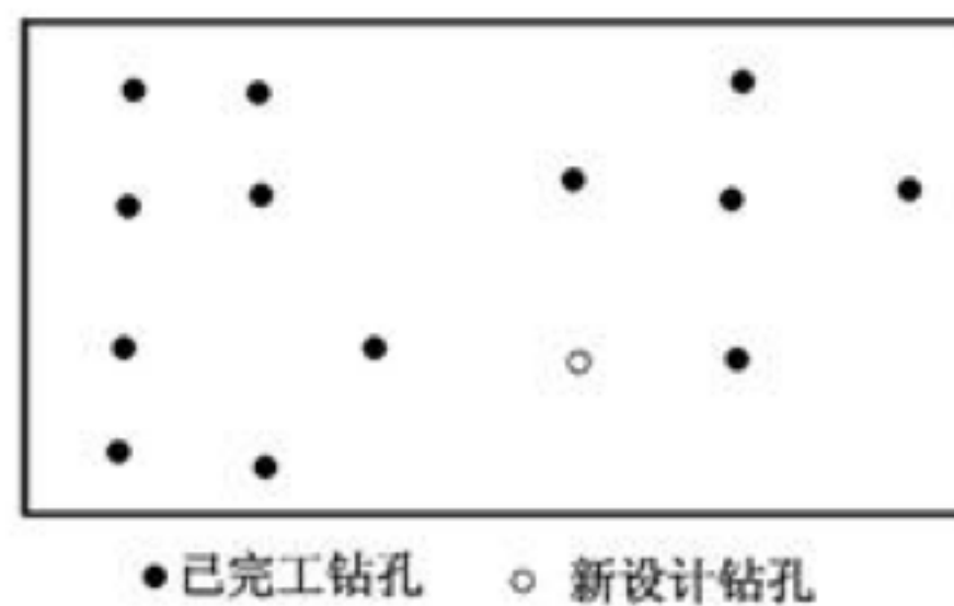
图 F.2 利用 \sigma_E^2 确定的最佳孔位
