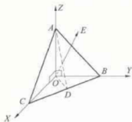
图 F.1 三面角反射器几何结构图
