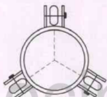
图 H. 2 滚轮式扶正器
