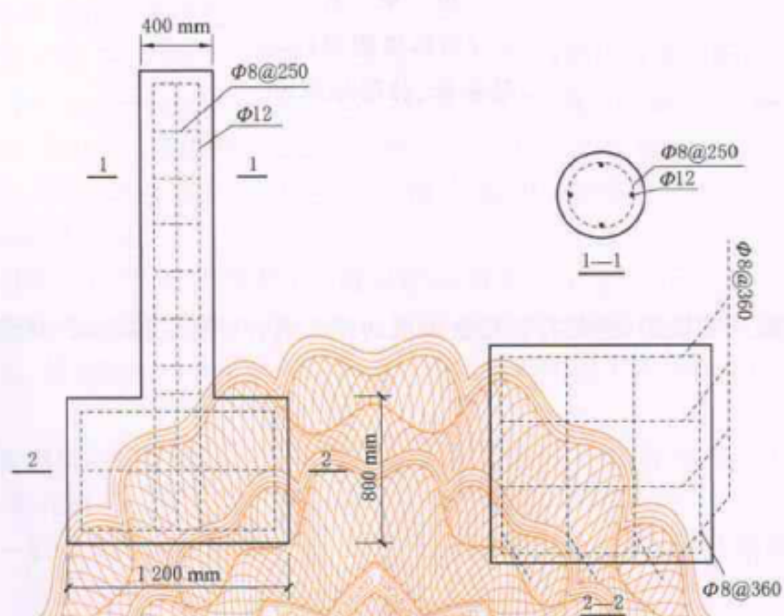
图 G.2 GPS 观测墩结构设计剖面图
