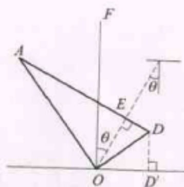
图 F.4 三面角反射器安装截面图定向示意图
