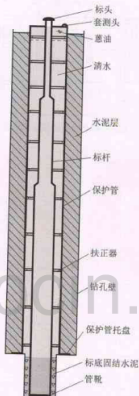
图 H.1 基岩标标型结构参考图
