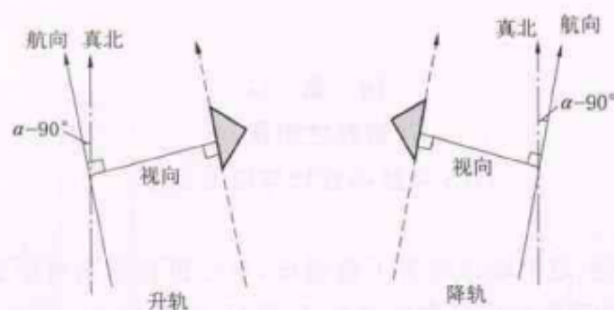
图 F.5 升、降轨模式下 CR 底边定向示意图
